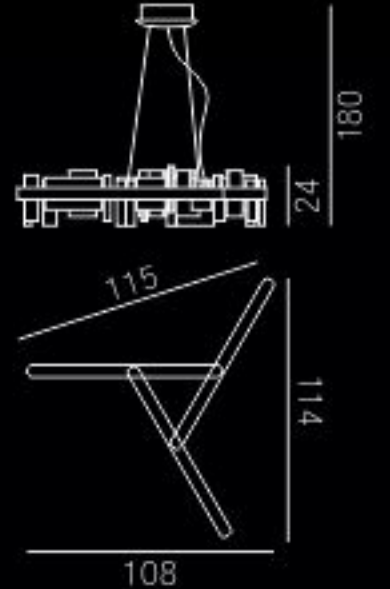
MD23057-1-1150 灯体尺寸: 115x108x180CM 功 率: LED 120W 材 质: 五金+云雾水晶 颜 色: 烤漆轻奢金
