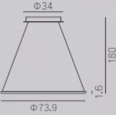
MD23051-1-750 灯体尺寸: \phi 73.9 \times 180\text{cm} 功 率: LED 46.8W 材 质: 五金+亚克力 颜 色: 亮光杏/卡其棕
