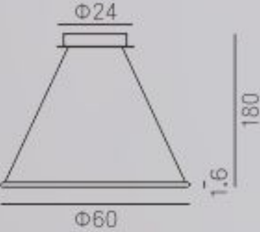
MD23051-1-600 灯体尺寸: \phi 60 \times 180\text{cm} 功 率: LED 37W 材 质: 五金+亚克力 颜 色: 亮光杏/卡其棕
