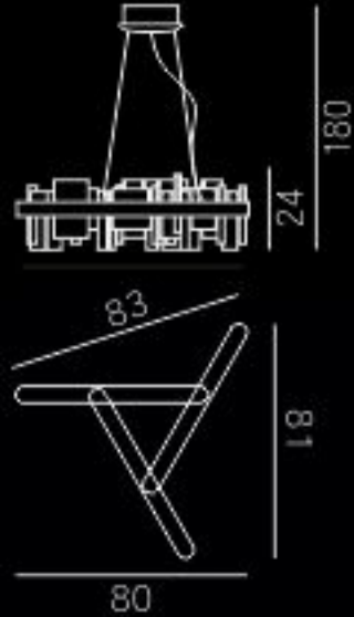
MD23057-1-830 灯体尺寸: 83x80x180CM 功 率: LED 90W 材 质: 五金+云雾水晶 颜 色: 烤漆轻奢金
