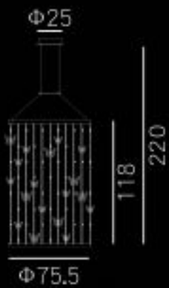
MD97241-2-755 灯体尺寸: \Phi 75.5 \times 220\text{CM} 功 率: LED 121.6W 材 质: 金属+蝴蝶水晶 颜 色: 哑白+幻彩
