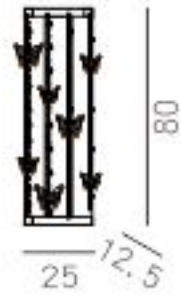
MB97241-1-250 灯体尺寸: 25×12.5×80CM 功 率: LED 7W 材 质: 金属+蝴蝶水晶 颜 色: 哑白+幻彩
