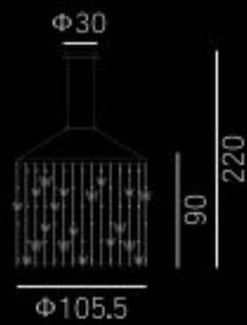
MD97241-2-1055 灯体尺寸: \Phi 105.5 \times 220\text{CM} 功 率: LED 167W 材 质: 金属+蝴蝶水晶 颜 色: 哑白+幻彩
